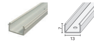
Монтажная планка Mounting strip
